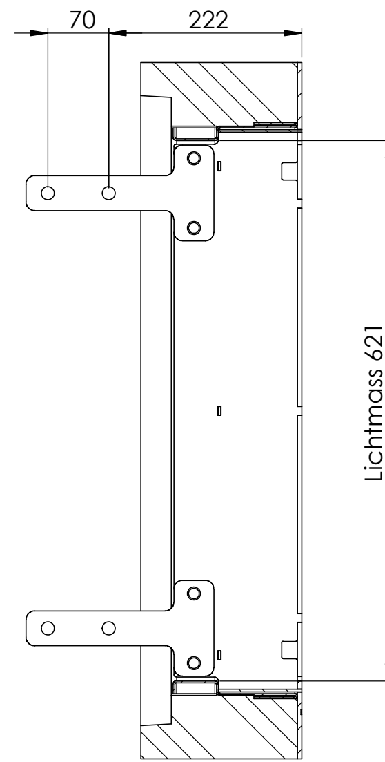
SCHNITT A-A
