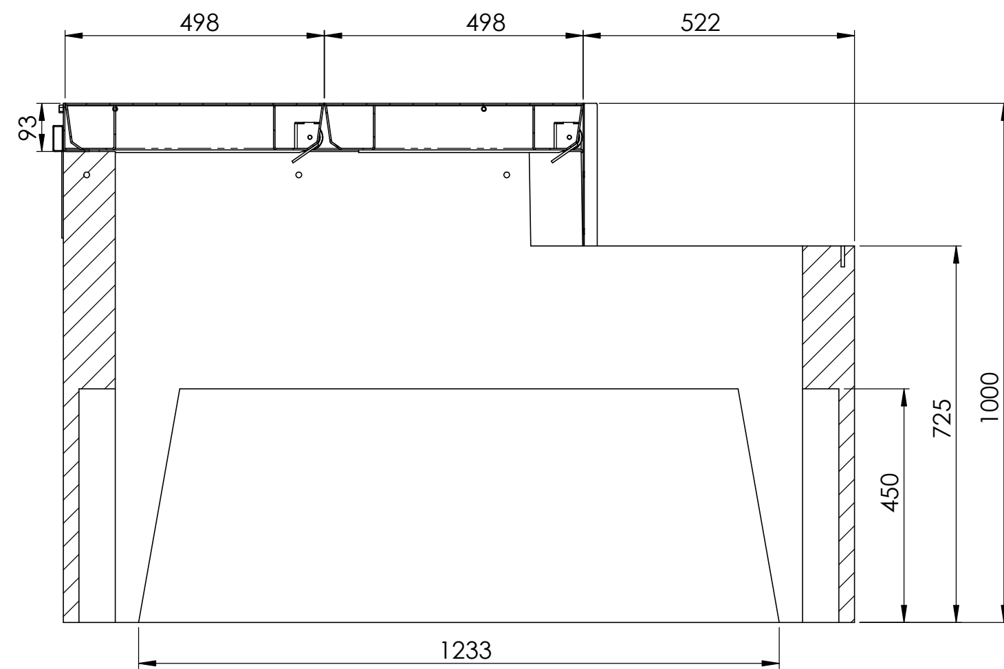
SCHNITT A-A
