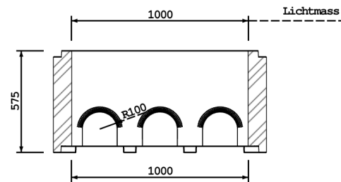
SCHNITT A-A
