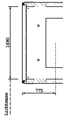
SCHNITT B-B
